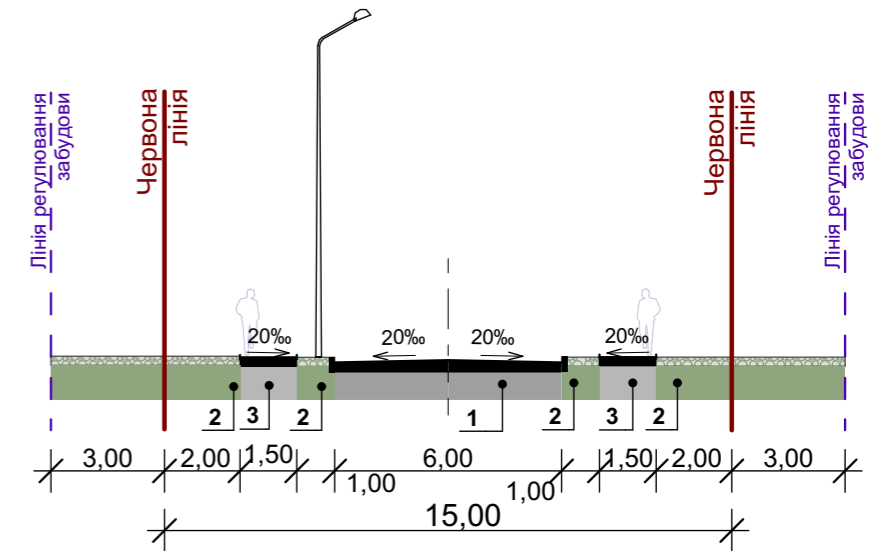
Поперечний профіль №3 вул. Проектна-1
