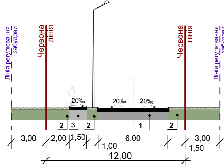
Поперечний профіль №4 проїзд Проектний-1
