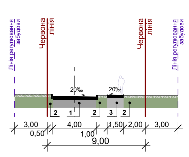
Поперечний профіль №7 проїзд Проектний-3
