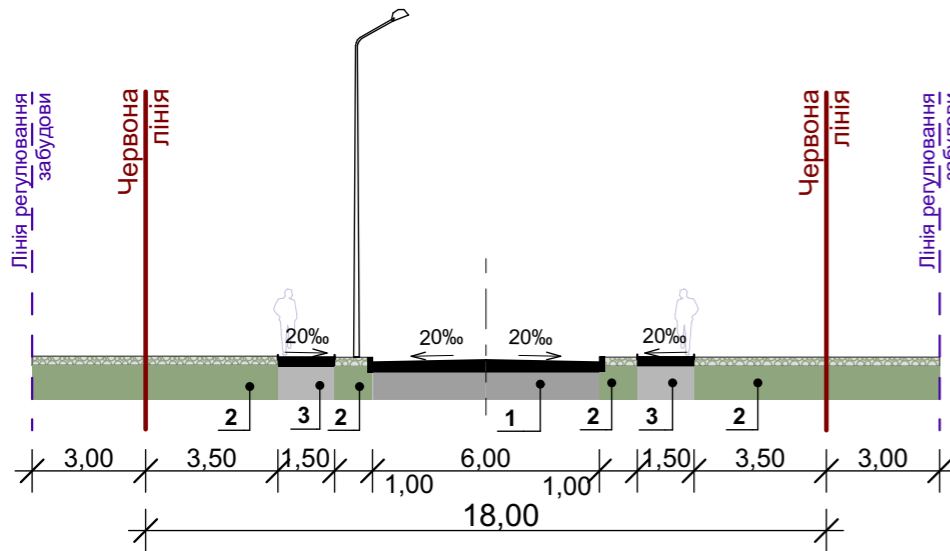
Поперечний профіль №1 вул. 8 Березня
