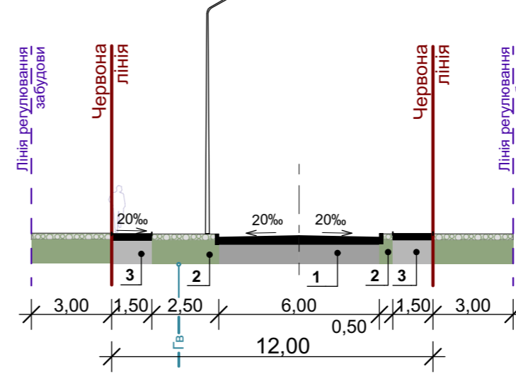
Поперечний профіль №6 вул. 8 Березня
