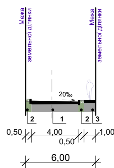
Поперечний профіль №5 проїзд Проектний-2
