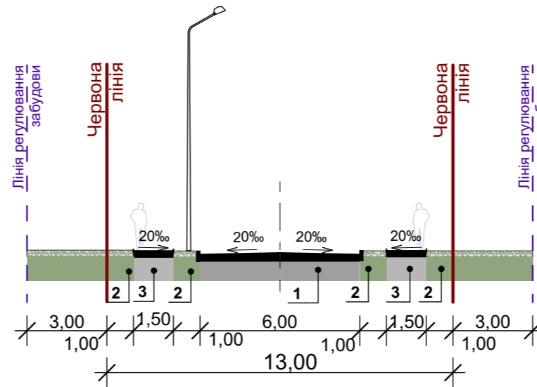
Поперечний профіль №2 вул. 8 Березня
